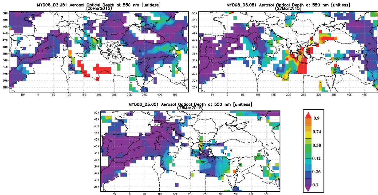
Şekil 7. MODIS-AOD ürünleri (26 - 28 Mart 2015)
