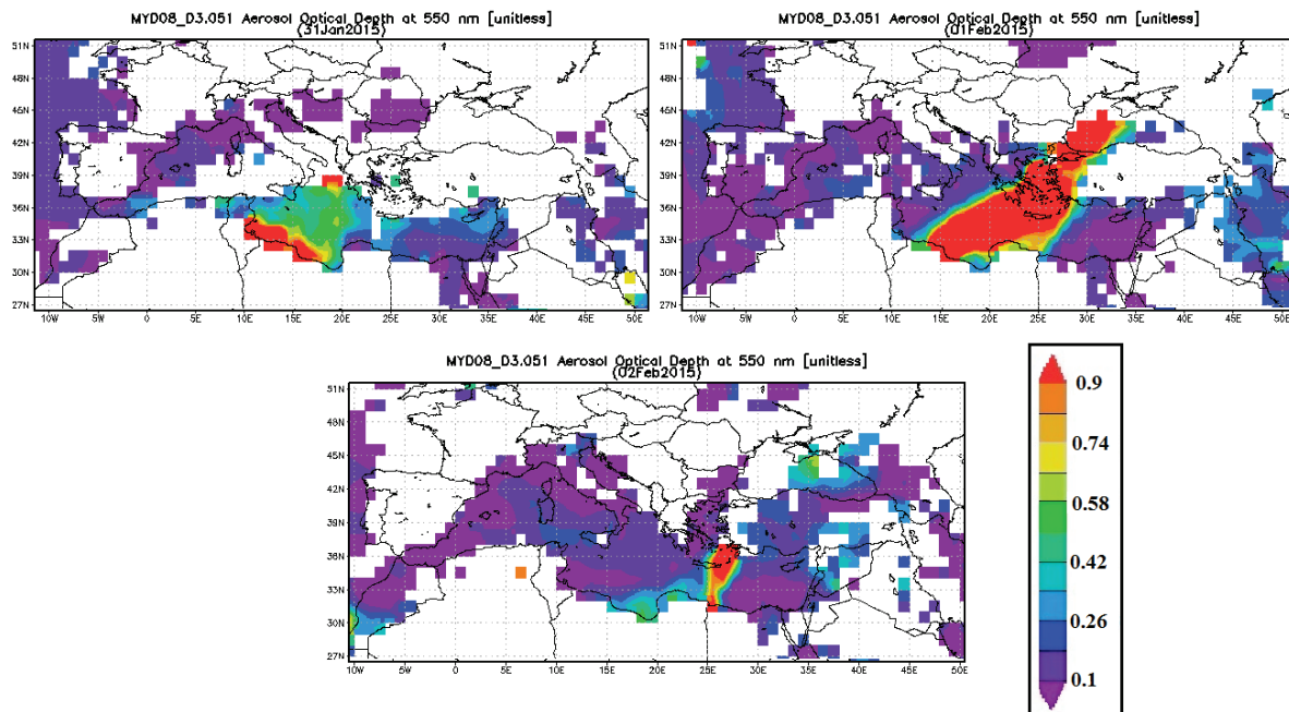
Şekil 3. MODIS-AOD ürünleri (31 Ocak - 2 Şubat 2015)
