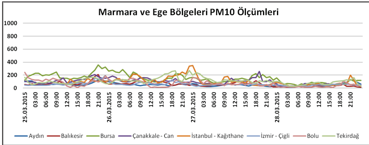
Şekil 5. Bazı şehirlerimizde ölçülen \text{PM}_{10} değerleri ( \mu\text{g}/\text{m}^3 ) (25 – 29 Mart 2015)
