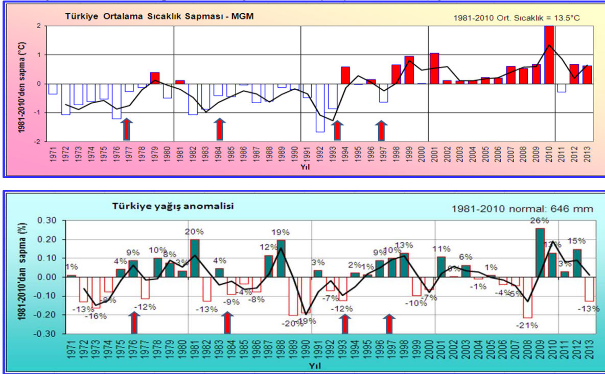
Şekil 4. Ortalama sıcaklık ve yağış anomaly grafikleri (1981-2010 normallerine göre).
