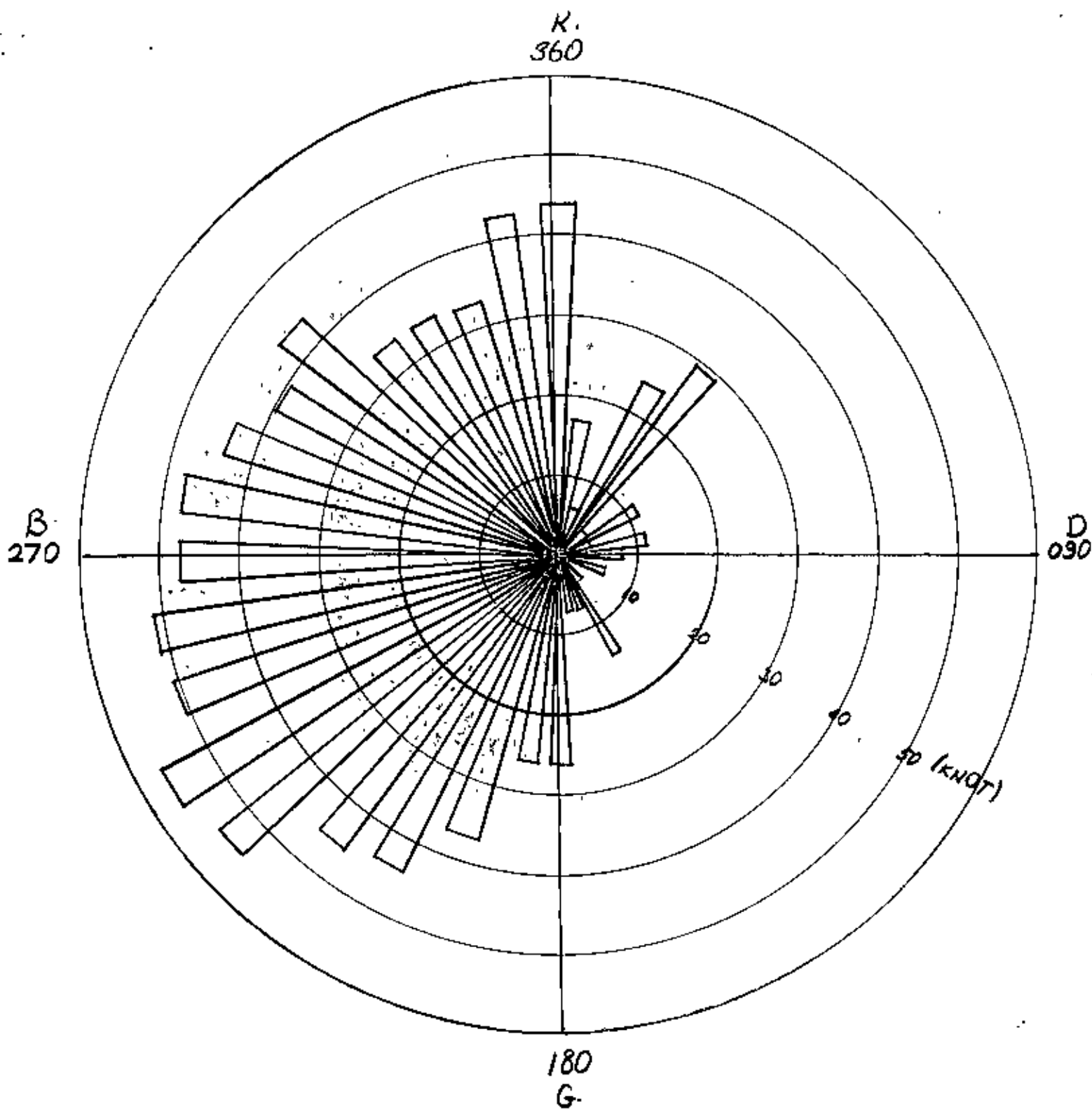
ANKARA 00° Z. SONBAHAR 200 MB HIZ ORTALAMASI
