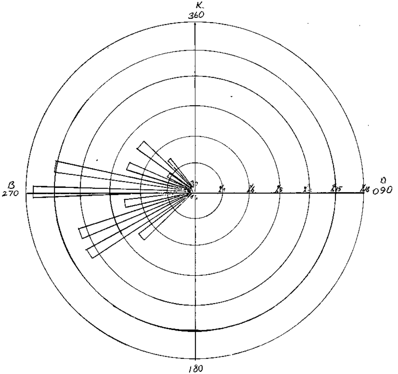
ANKARA 00° Z. ARALIK AYI 50 MB. FREKANS YÜZDESİ
