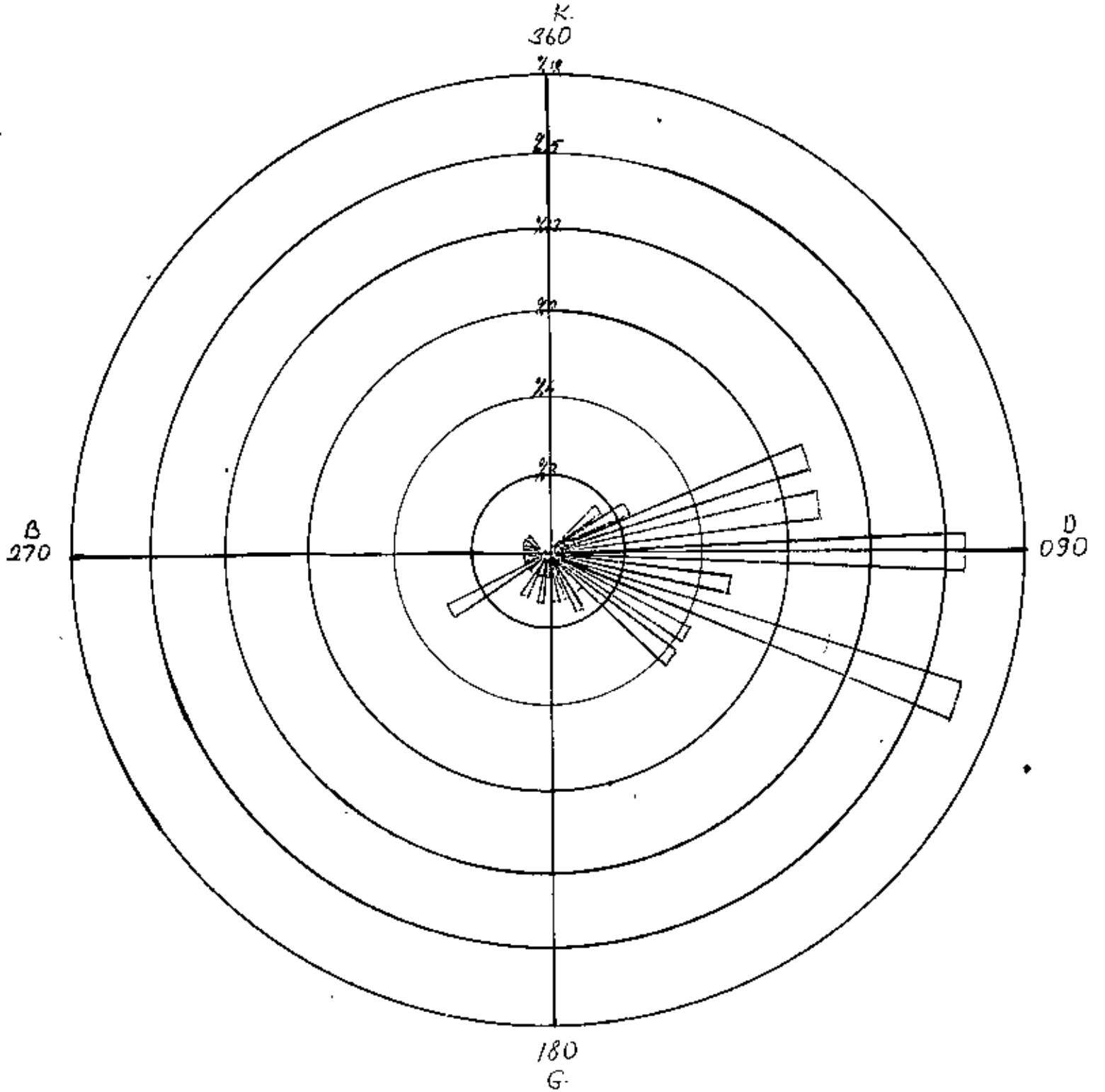
ANKARA 00°Z. TEMMUZ AYI 50 MB. FREKANS YÜZDESİ
