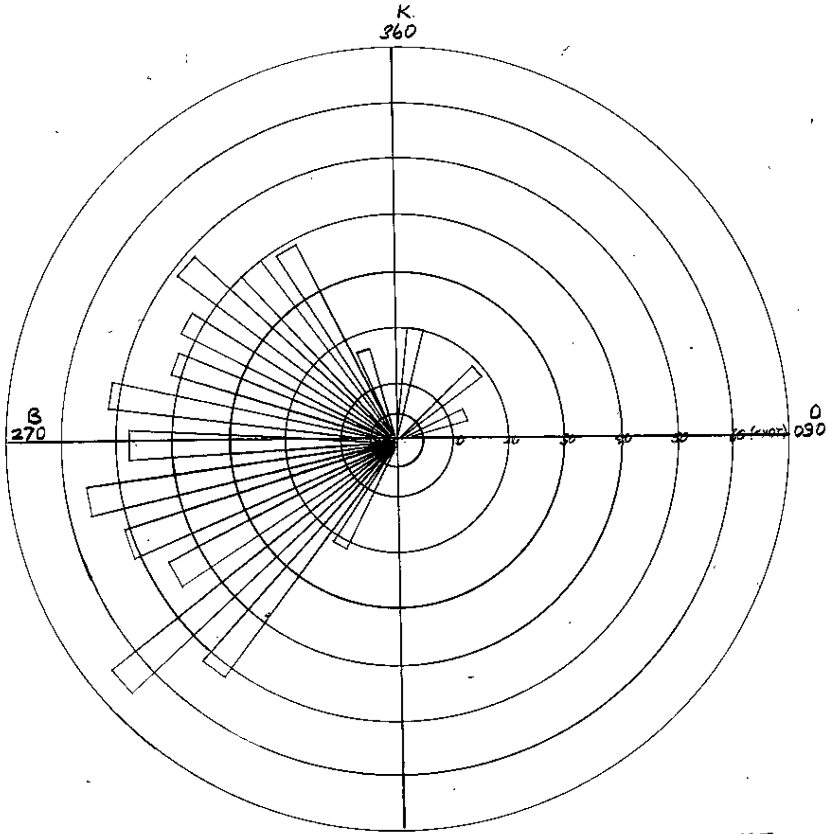
ANKARA 00°Z. ARALIK AYI 100 MB. HIZ ORTALAMASI
