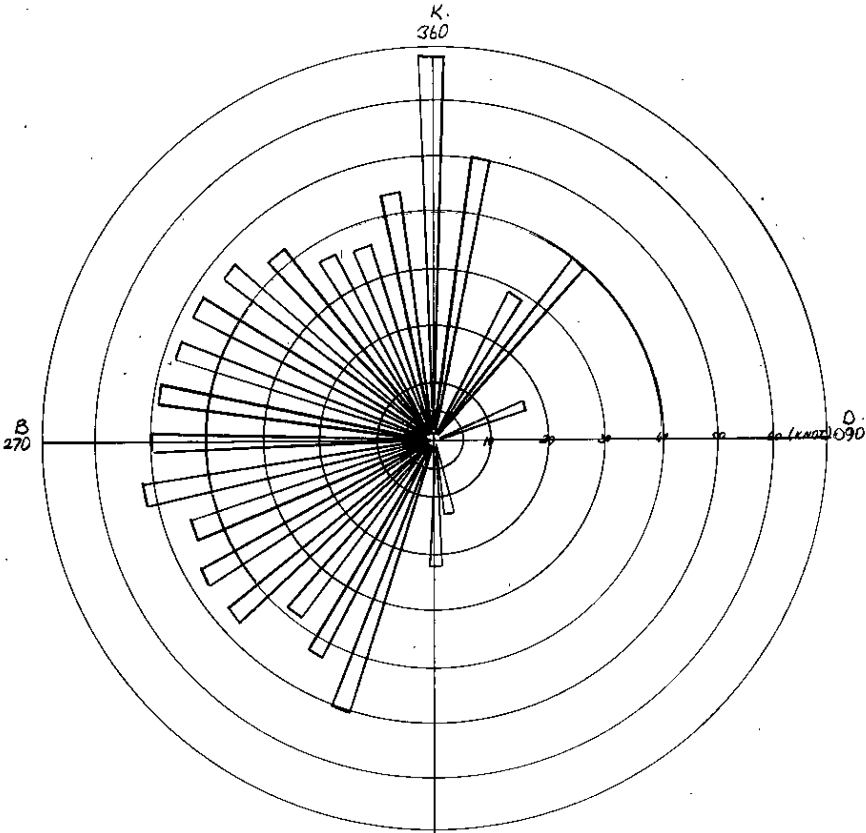
ANKARA 00°Z. KASIM AYI 200 MB. HIZ ORTALAMASI
