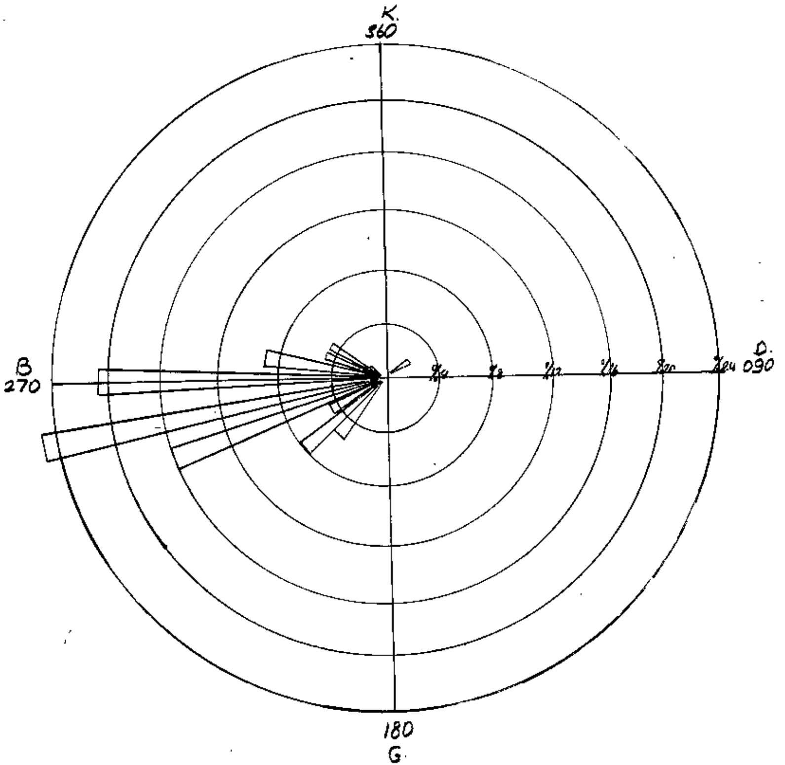
ANKARA 00 00 Z- MART AYI 50 MB. FREKANS YÜZDESİ
