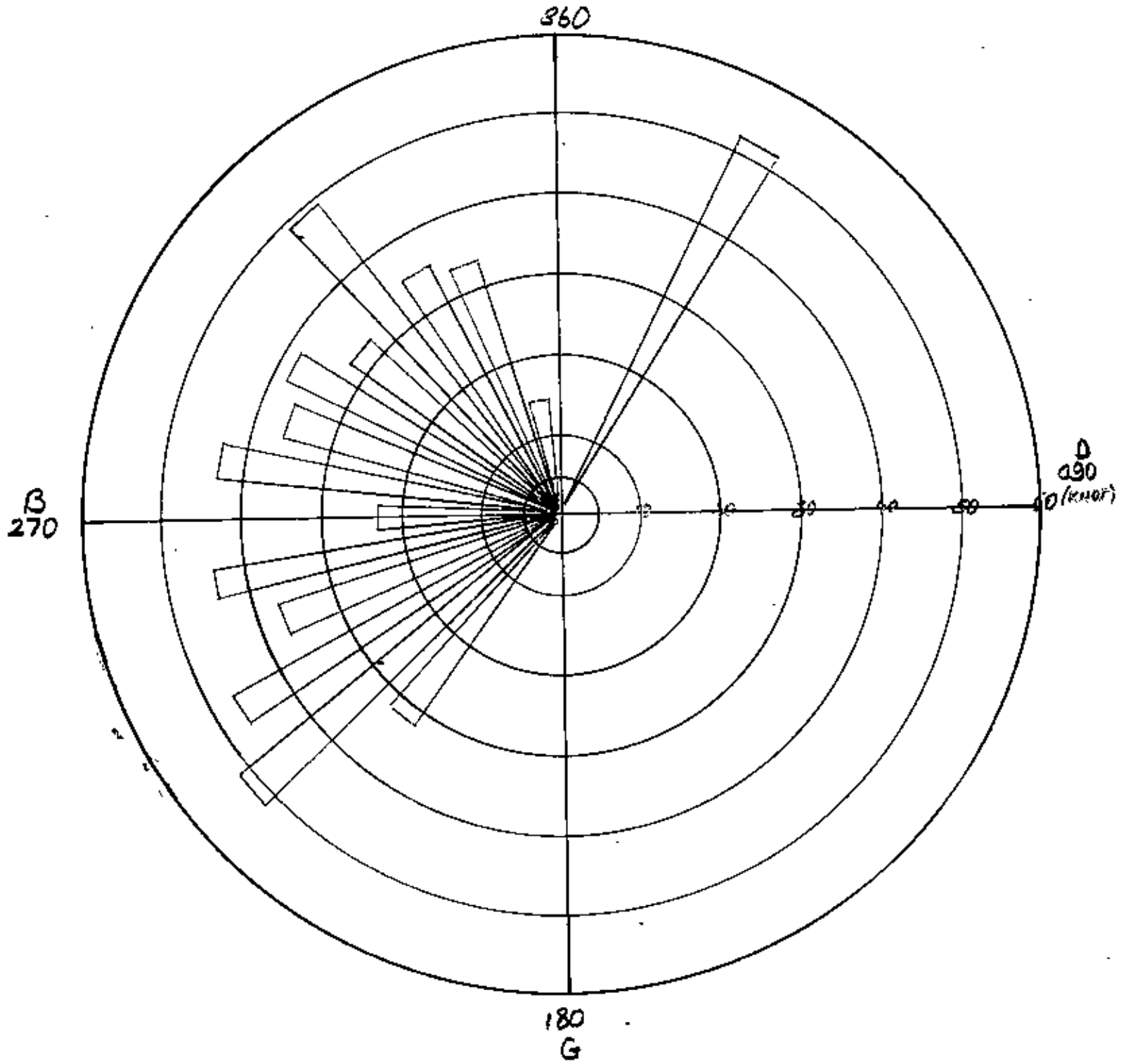
ANKARA 00°Z. KASIM AYI 100 MB. HIZ ORTALAMASI
