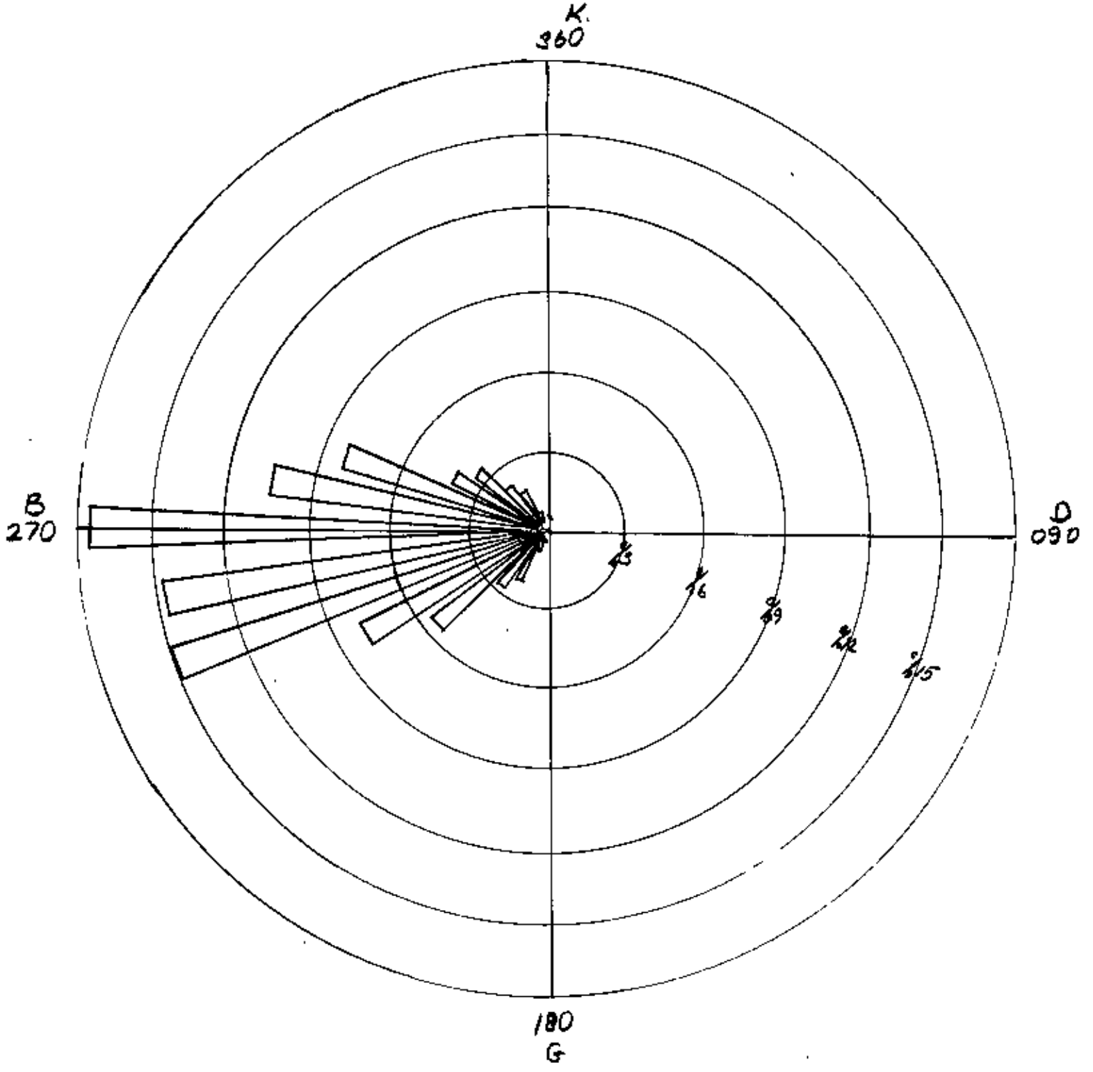
ANKARA 00° Z SONBAHAR 100 MB. FREKANS YÜZDESİ
