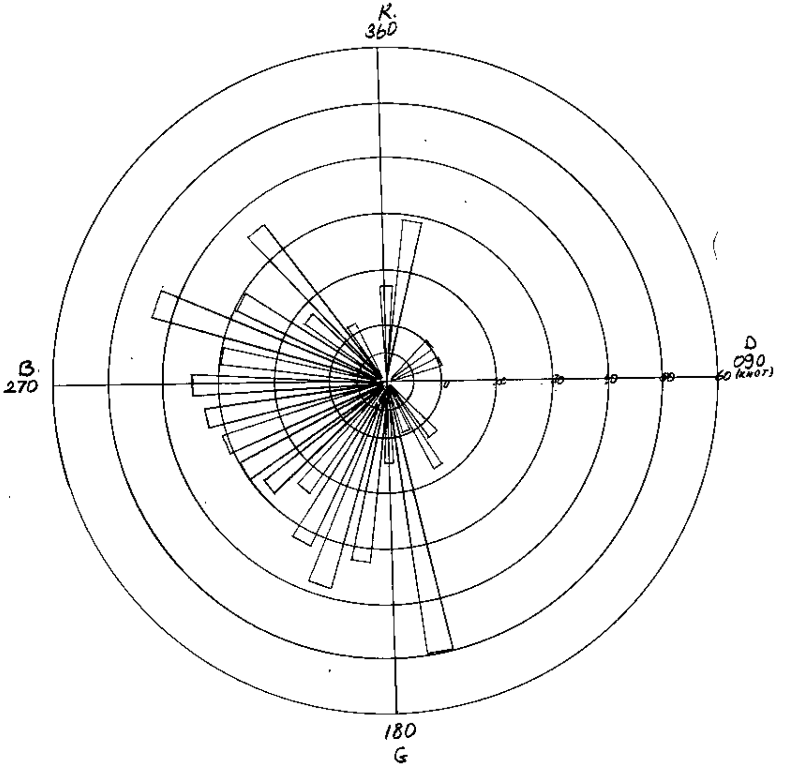
ANKARA 00°Z. MAYIS AYI 100 MB. HIZ ORTALAMASI
