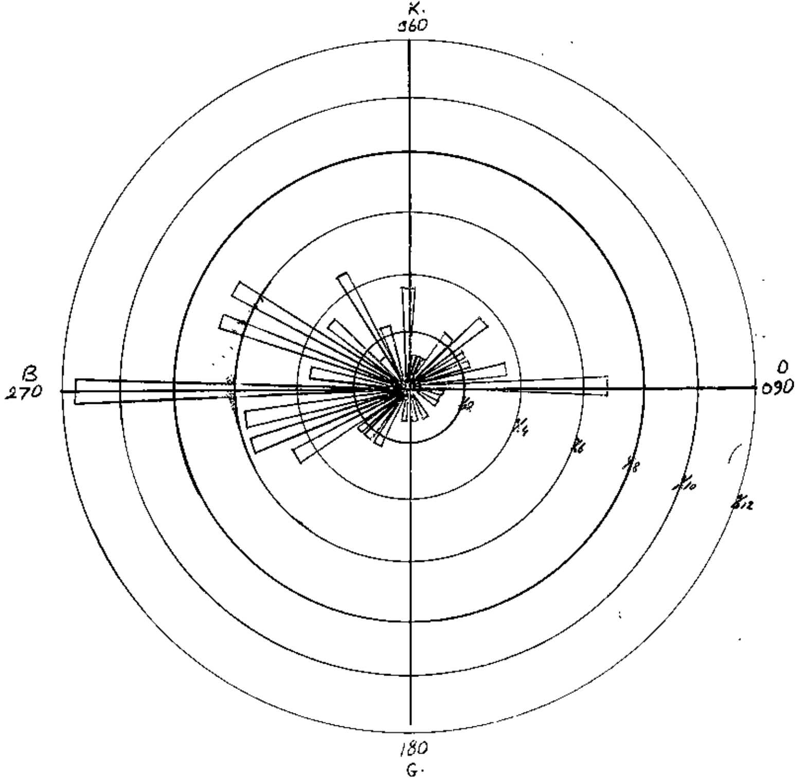
ANKARA 00°Z. EYLÜL AYI 50 MB. FREKANS YÜZDESİ
