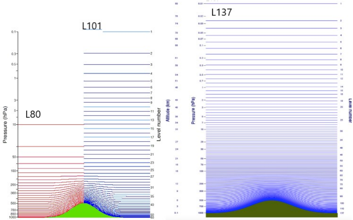
řekil 3- Atmosfer modelinde sigma koordinatlarında kullanılan model seviyeleri.
