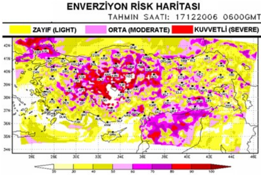
Şekil-6, ECMWF model verilerinden elde enverziyon tahmin haritası.
